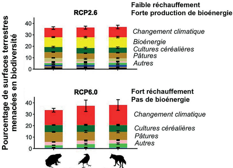
Figure 6.8 : Pourcentage de surfaces terrestres qui risquent d'être perdues pour la biodiversité des amphibiens, des oiseaux et des mammifères selon deux scénarios . Dans la figure du bas ( scénario sans production de bioénergie ), l'impact dominant sur la biodiversité est le changement climatique, car l'utilisation des énergies fossiles conduit à des émissions élevées de gaz à effet de serre et à un fort réchauffement de la planète. Dans la figure du haut ( scénario avec production massive de bioénergie ), l'impact associé à l'utilisation de grands espaces pour les plantations « énergétiques » est de même ampleur que l'impact dû au changement climatique. Source : [6] CC BY-NC-ND 4.0.
