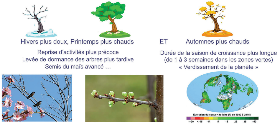
Figure 8.5: Influence du réchauffement climatique sur la végétation (Source : Nathalie de Noblet-Ducoudré). Verdississement de la planète (Source : Boston University / Ranga Myneni).
