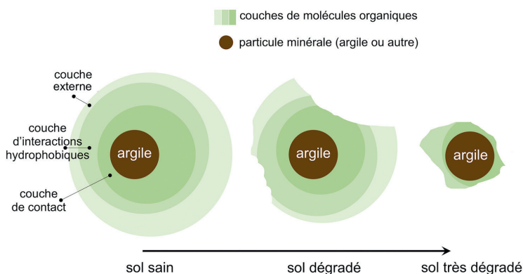
Figure 2.28 : Structure multicouche associant une particule d'argile et des molécules organiques riches en carbone, selon le modèle de Kleber [16] . La réduction des couches organiques, externes, intermédiaires, voire de contact, conduit à des sols de plus en plus dégradés (de gauche à droite). Source : Christine Hatté
