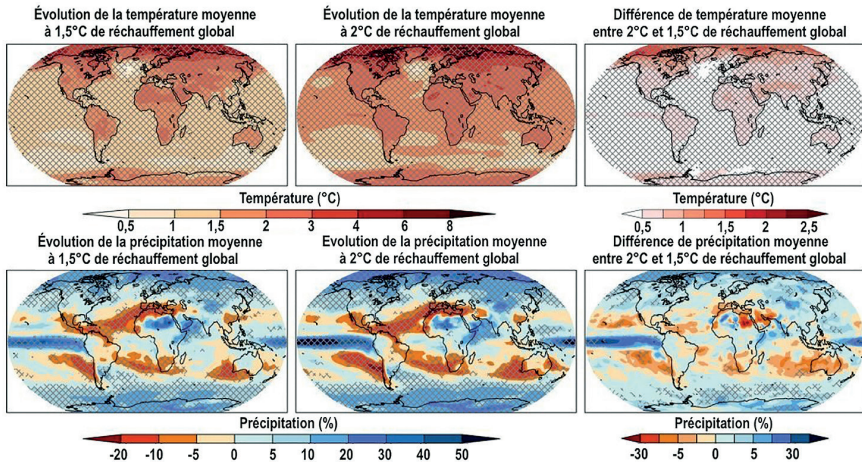
Figure 8.4 : Projection des changements de température moyenne (en haut) et de précipitations moyennes (en bas) pour un réchauffement moyen planétaire de 1,5 °C (à gauche) et 2 °C (au milieu) en prenant pour référence la période préindustrielle (1861-1880). Les zones hachurées représentent les zones où plus de deux tiers des modèles (au moins 18 sur 26) s'accordent sur le signe du changement et sont donc les zones où les résultats sont considérés comme robustes. Source : SRI.5 IPCC, Chapitre 3 72 .
