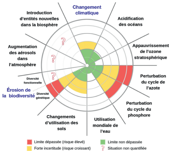
Figure 1 : Enjeux planétaires globaux. Le concept des limites planétaires définit un espace de développement sûr et juste pour l'humanité, fondé actuellement sur neuf [1] processus biophysiques. Des seuils quantitatifs ont été définis pour sept des neuf limites. En 2009, J. Rockström indiquait que trois d'entre elles étaient franchies (changement climatique, érosion de la biodiversité, perturbation du cycle de l'azote). Lors de la révision du modèle conceptuel [2], de nouveaux seuils ont pris en compte le niveau régional et l'hétérogénéité des processus. En dépit de débats encore suscités à ce sujet, le concept est reconnu et adopté aux niveaux européen et international. Figure adaptée de [2].
